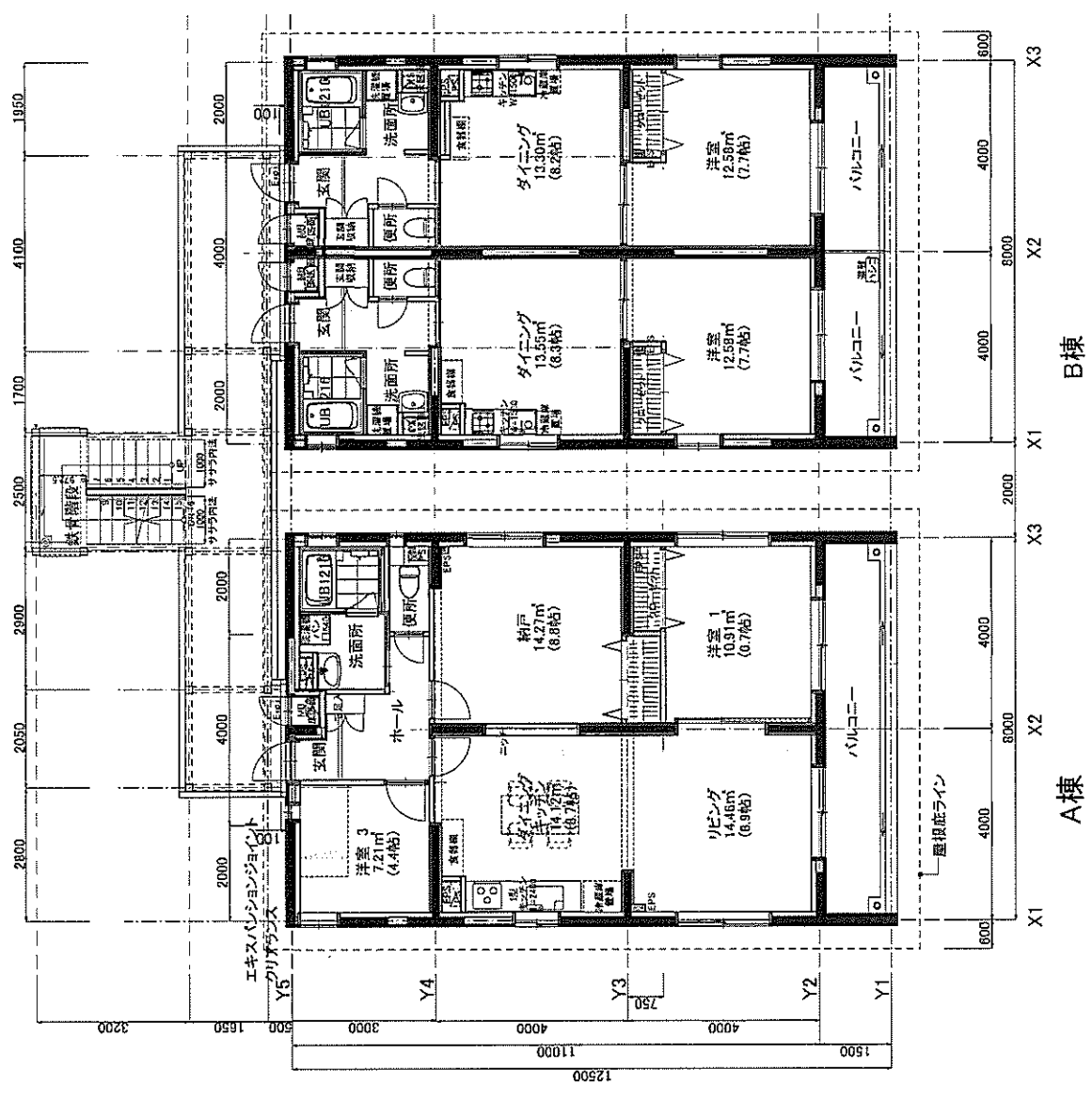
2階平面図 1/100
