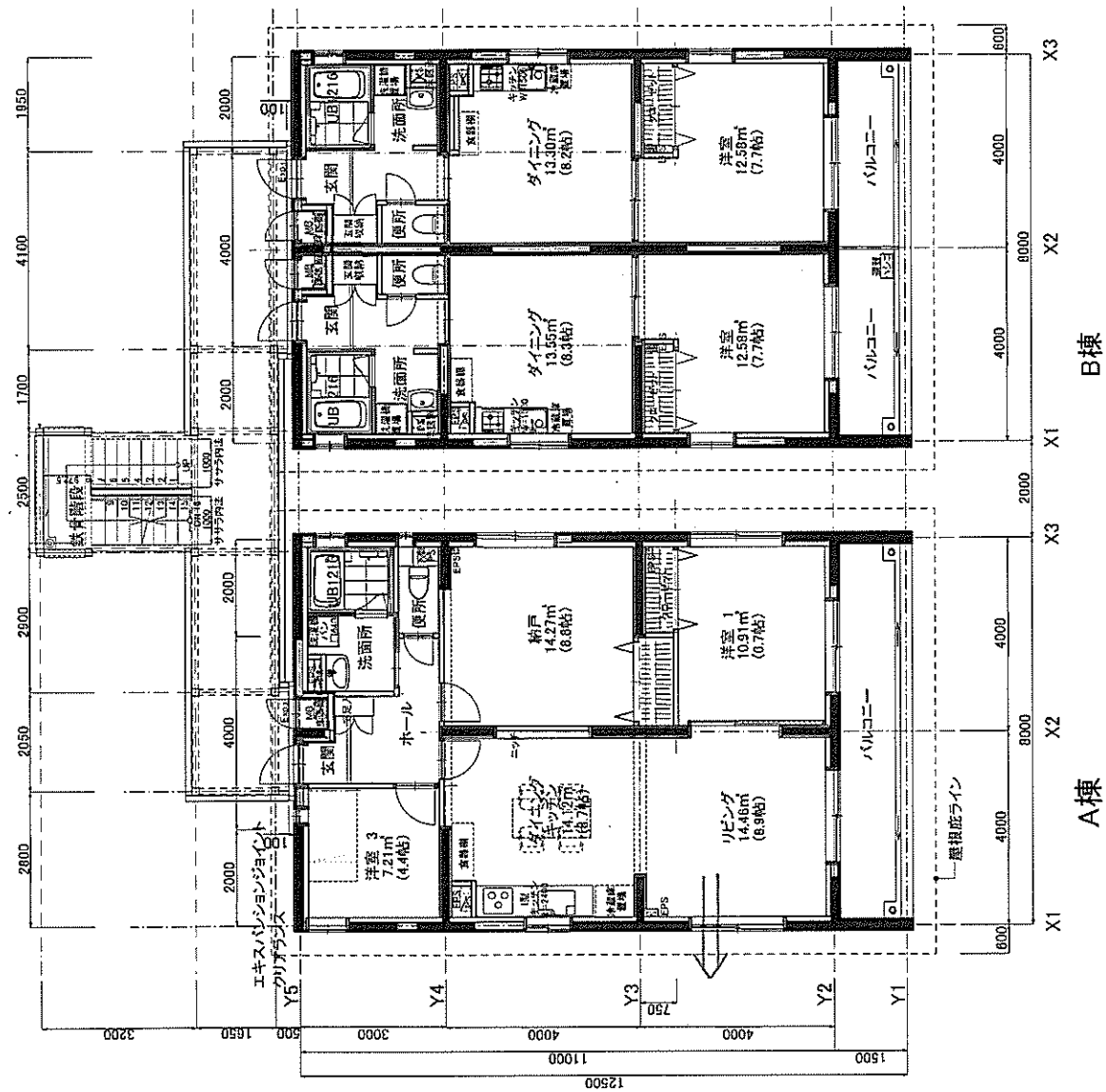
2階平面図 1/100
