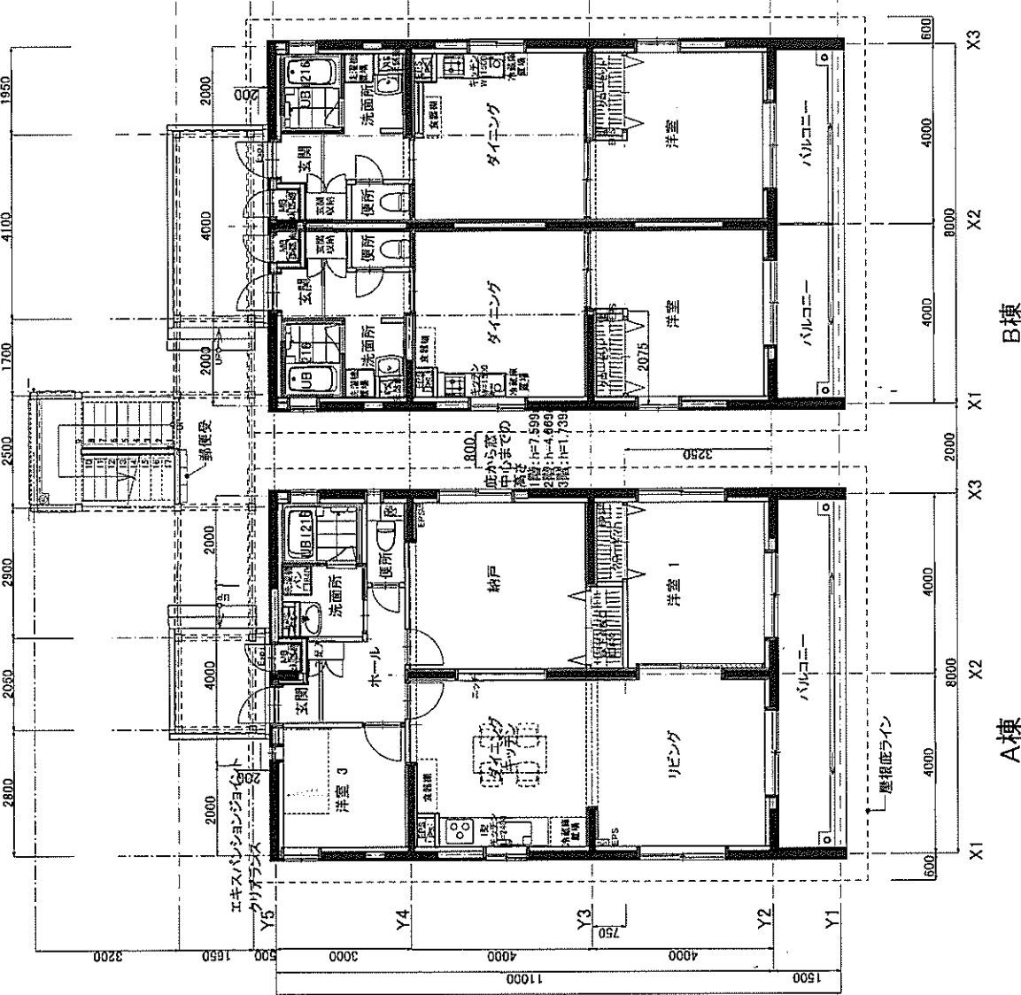
1階平面図 1/100
