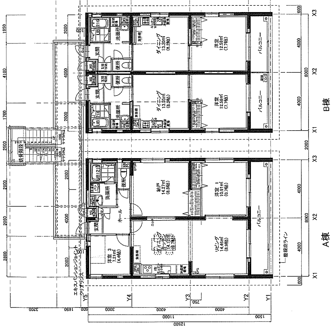
2階平面図 1/100
