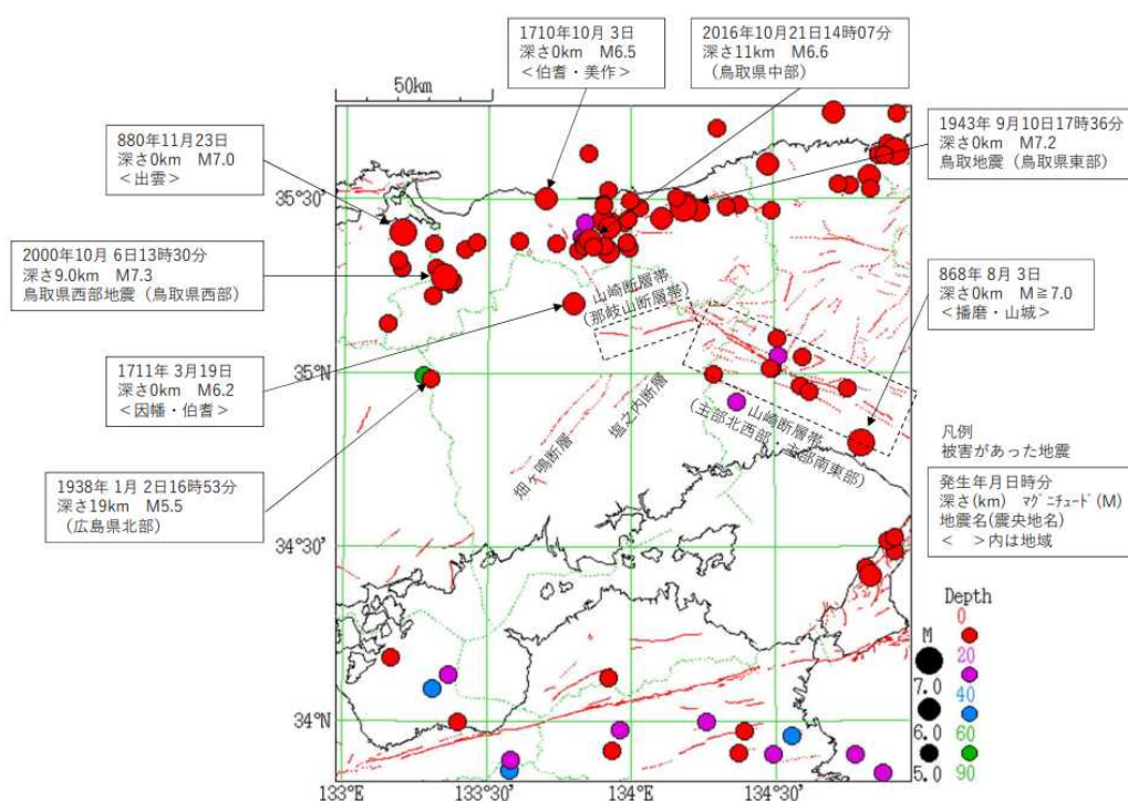
図2 岡山県とその周辺の地震活動（601年1月1日～2023年12月31日M5.0以上）
