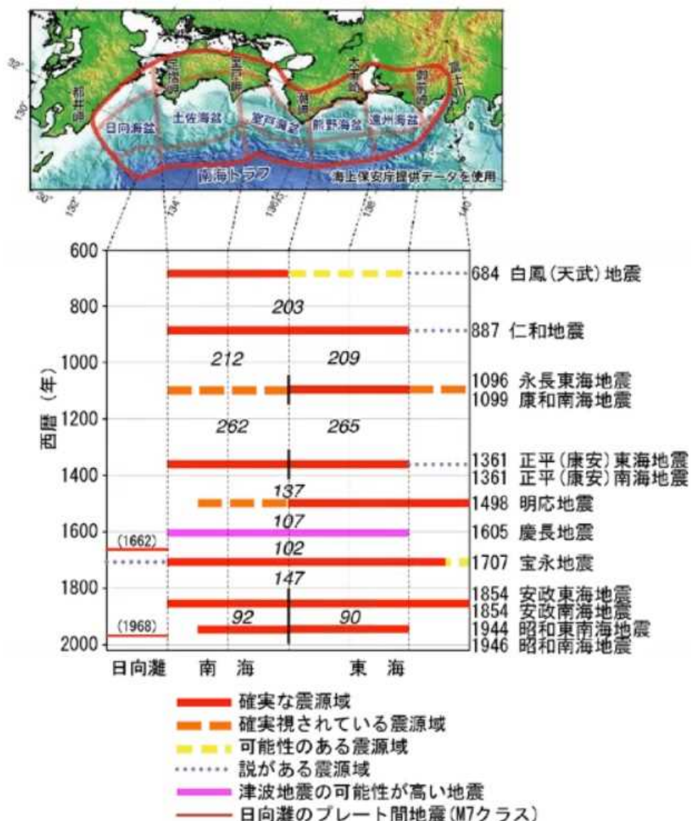
図3 南海トラフ—駿河トラフ沿いの過去の巨大地震
