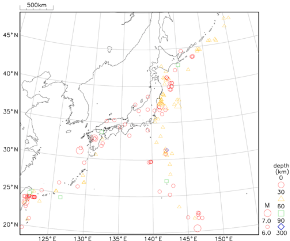
図1 日本及び周辺の最近10年の地震活動（平成26年～令和5年、M6.0以上）
