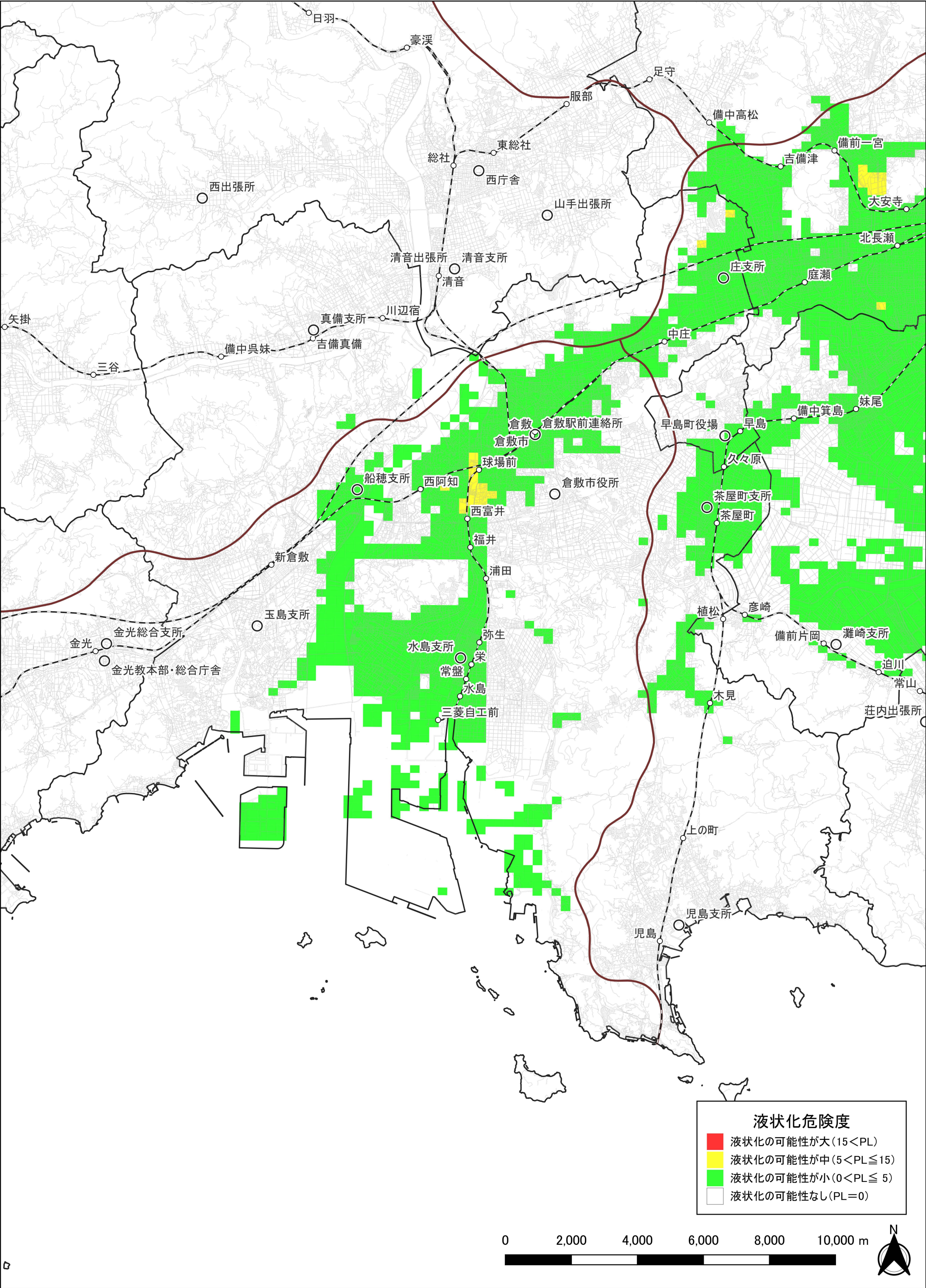
山崎断層帯主部の地震による液状化危険度分布図【岡山県想定（2025年度）】 倉敷市
