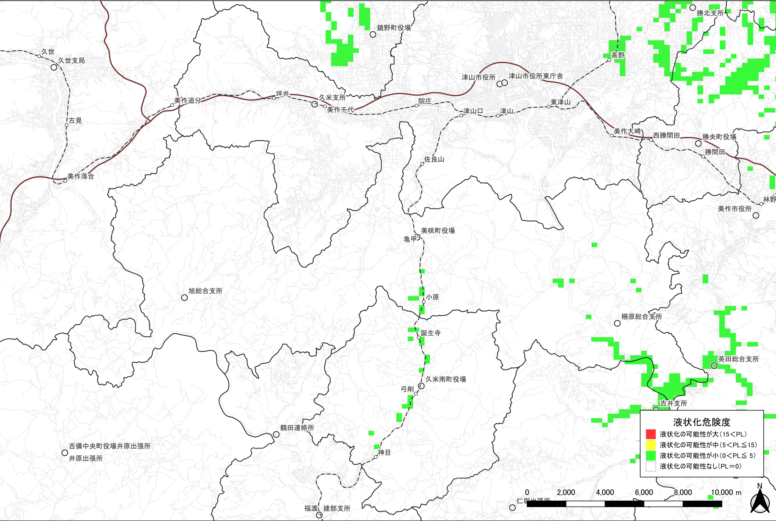
山崎断層帯主部の地震による液状化危険度分布図【岡山県想定（2025年度）】 美咲町
