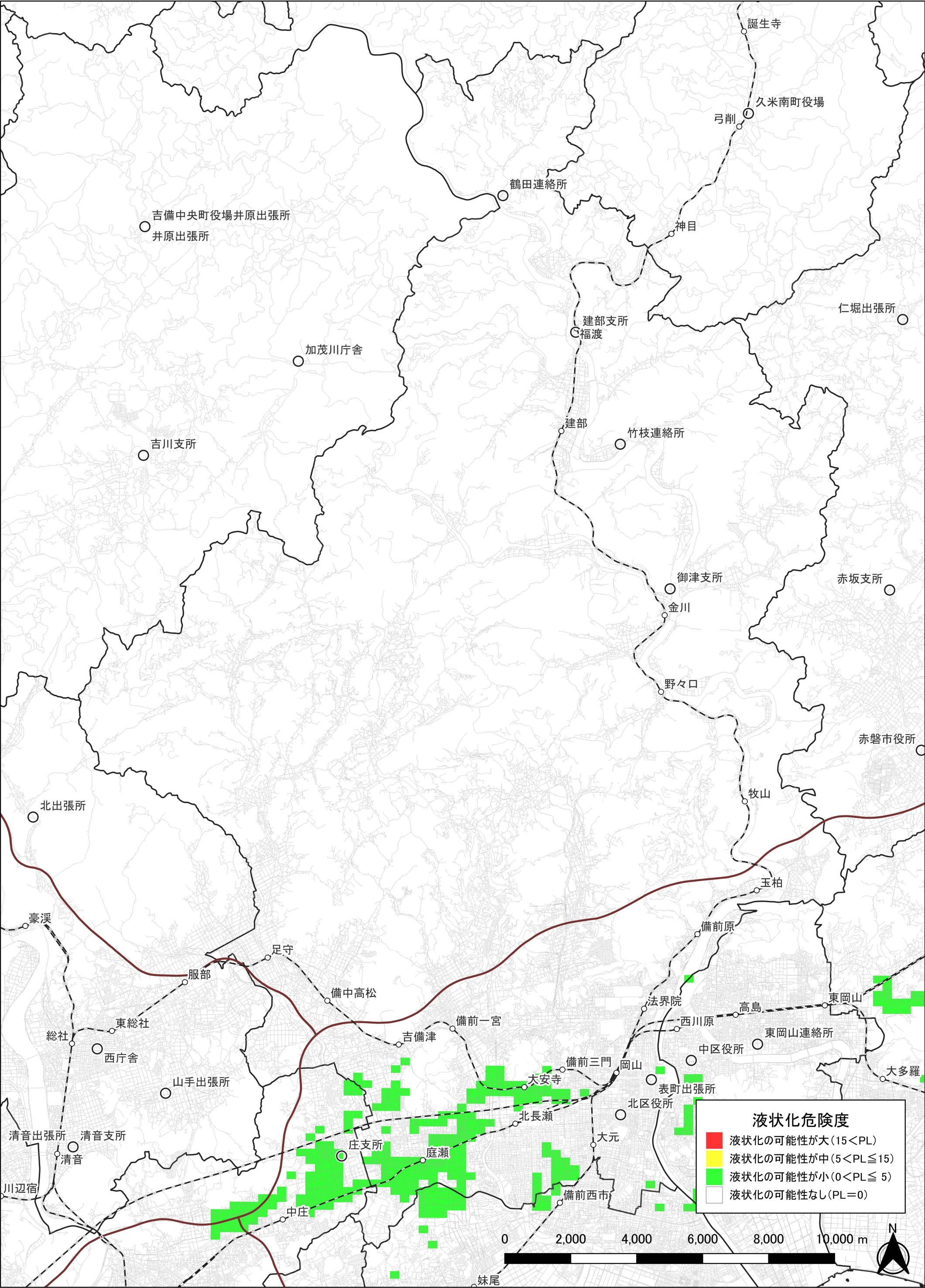
那岐山断層帯の地震による液状化危険度分布図【岡山県想定（2025年度）】 岡山市北区
