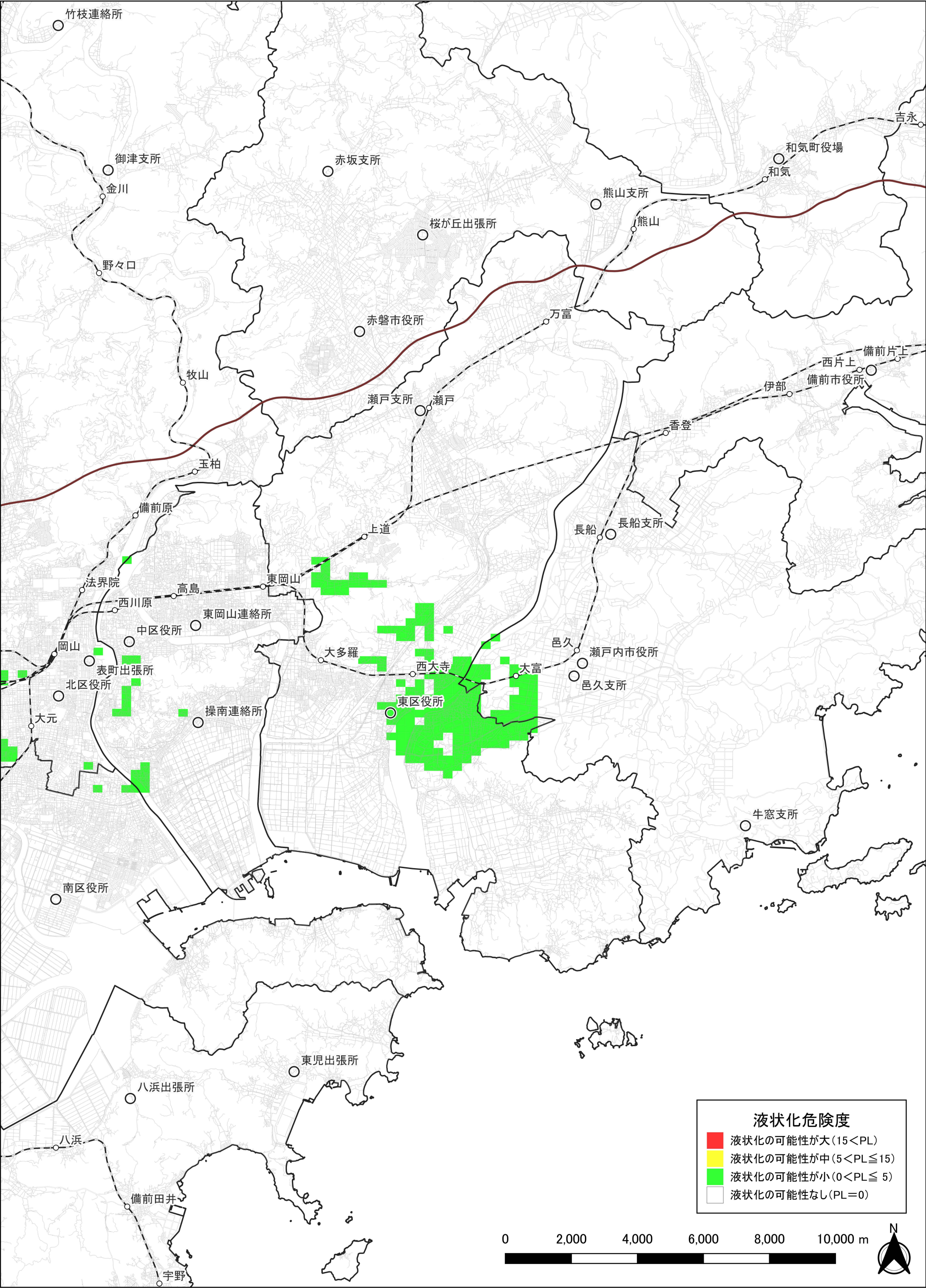
那岐山断層帯の地震による液状化危険度分布図【岡山県想定（2025年度）】 岡山市東区
