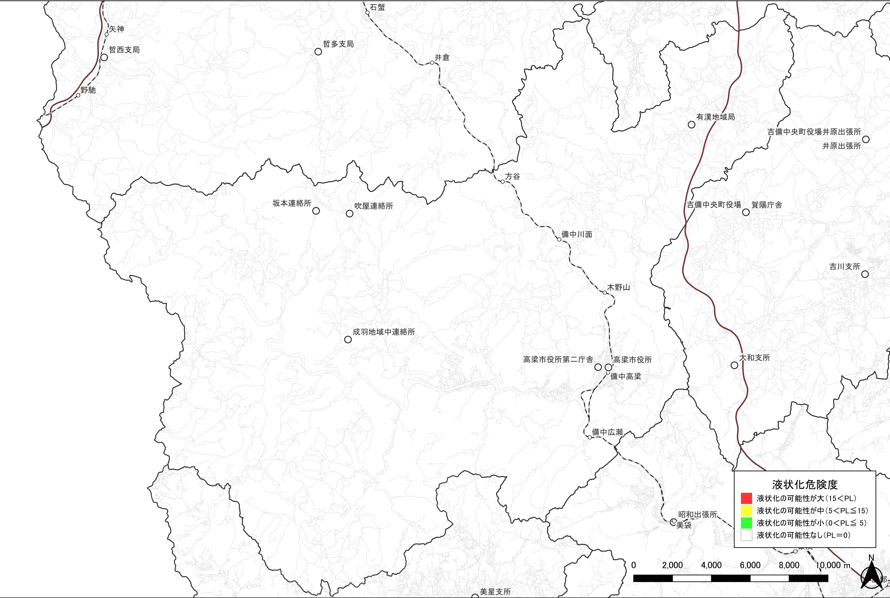
那岐山断層帯の地震による液状化危険度分布図【岡山県想定（2025年度）】 高梁市
