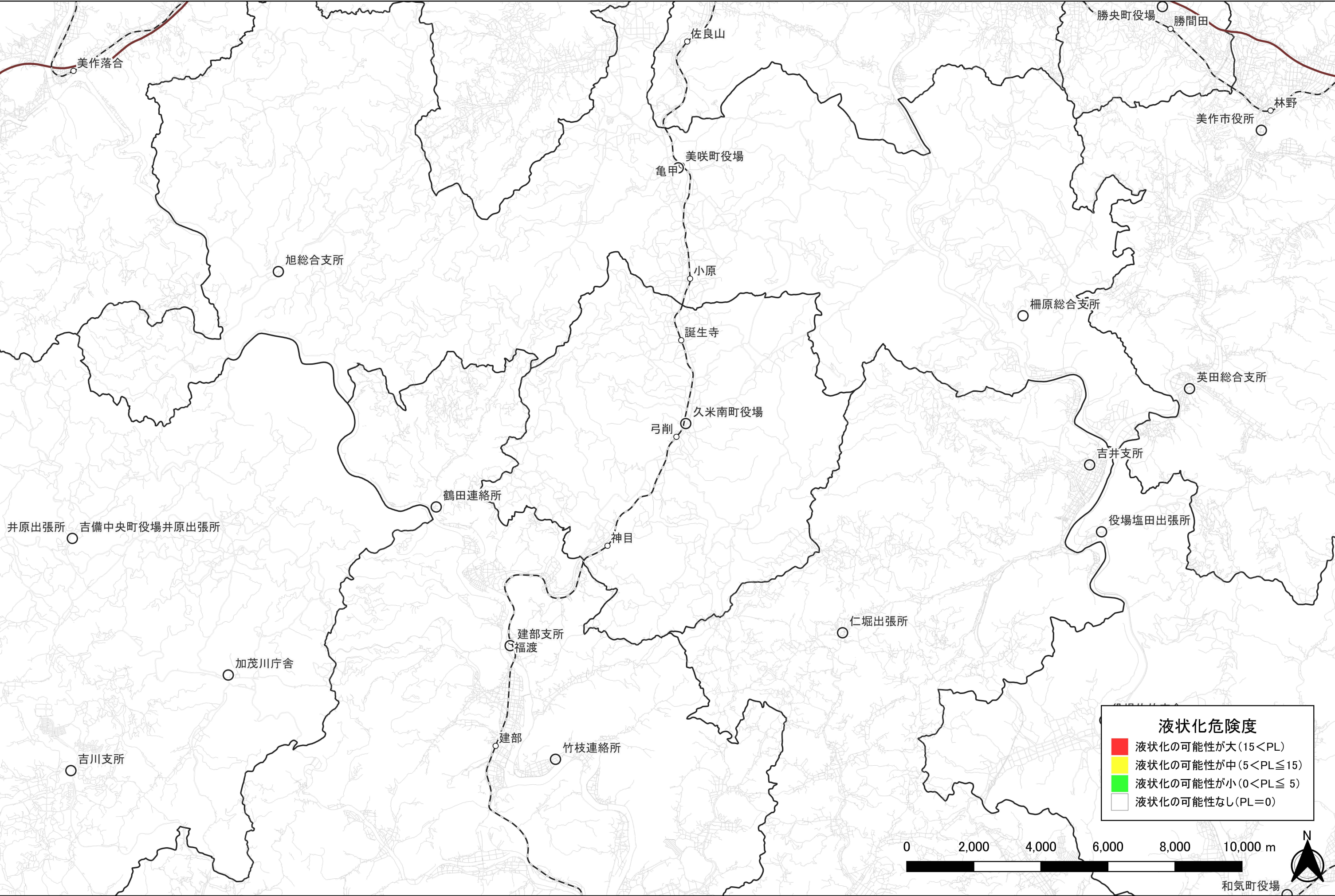
那岐山断層帯の地震による液状化危険度分布図【岡山県想定（2025年度）】 久米南町
