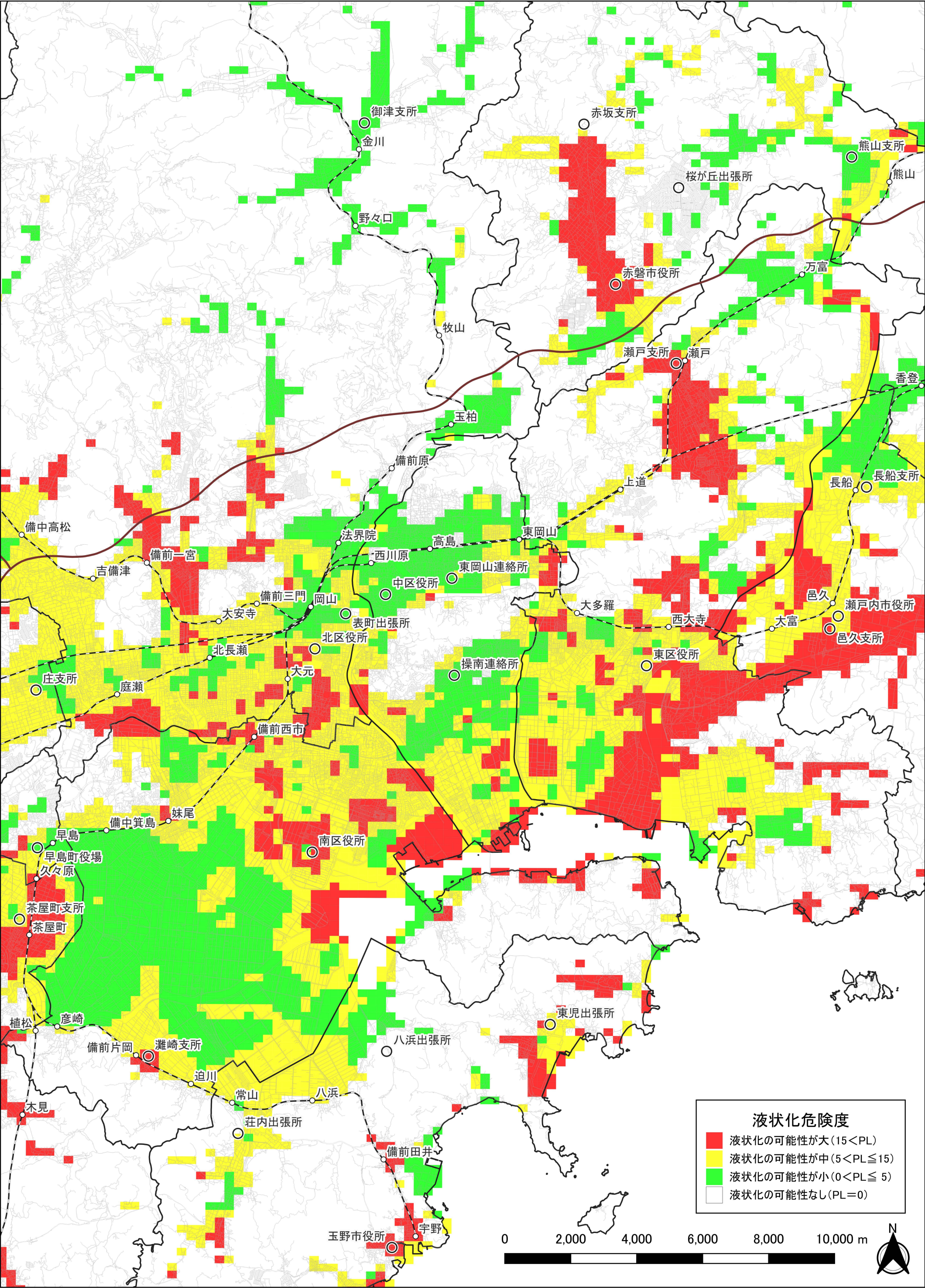
南海トラフ巨大地震による液状化危険度分布図【岡山県想定（2025年度）】 岡山市中区
