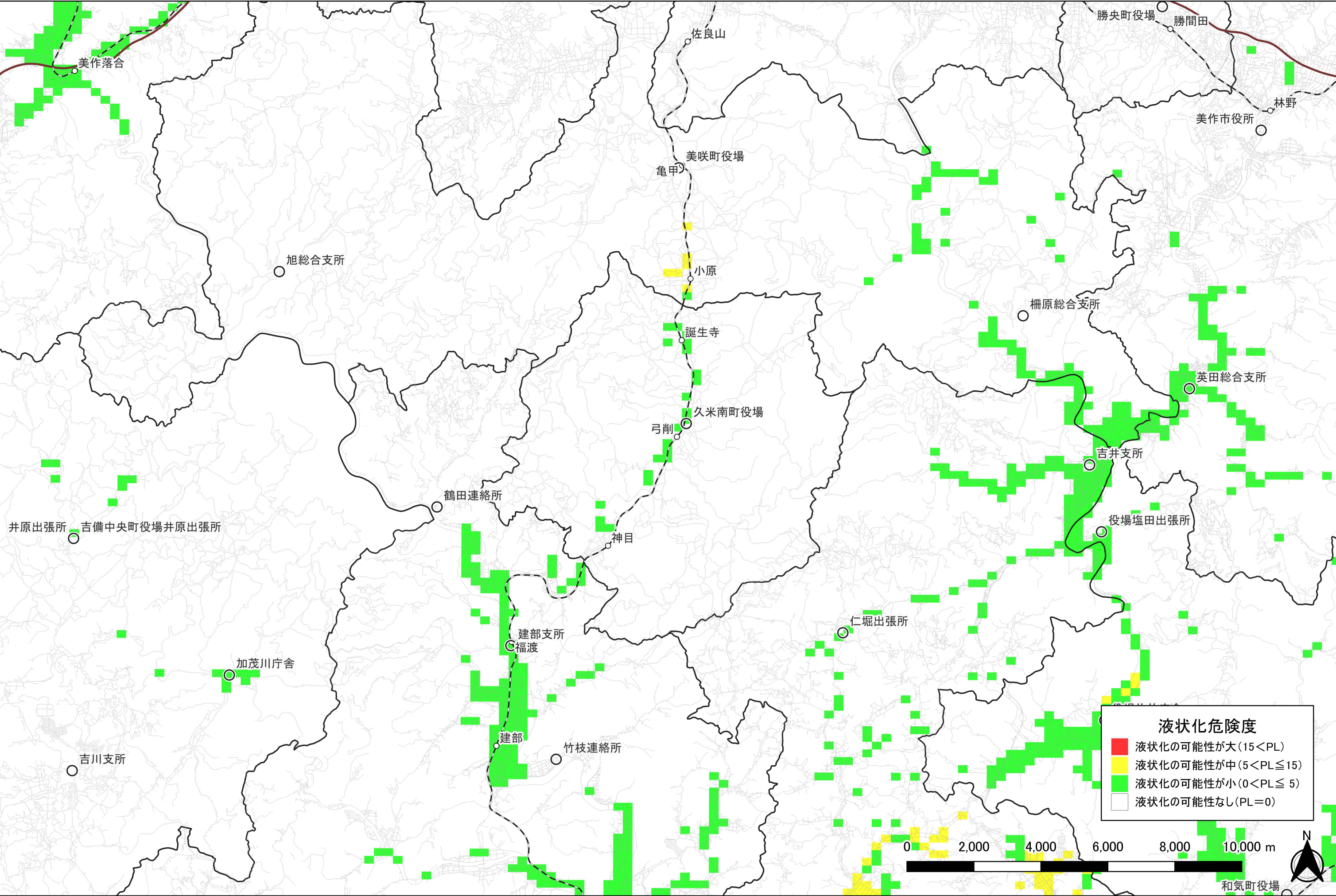
南海トラフ巨大地震による液状化危険度分布図【岡山県想定（2025年度）】 久米南町
