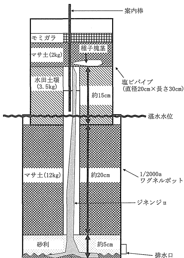
図1 ポットを用いた再現試験法
