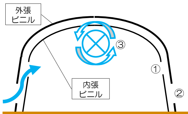
図1 側窓優先換気ハウス
