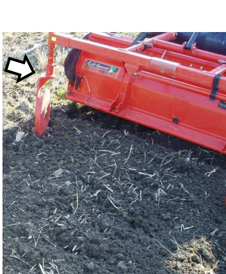
図4 尾輪の装着（矢印）
