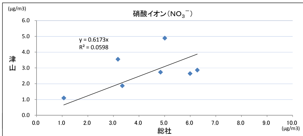
図11-2 (H25 冬季) 総社と津山における硝酸イオンの測定値比較
