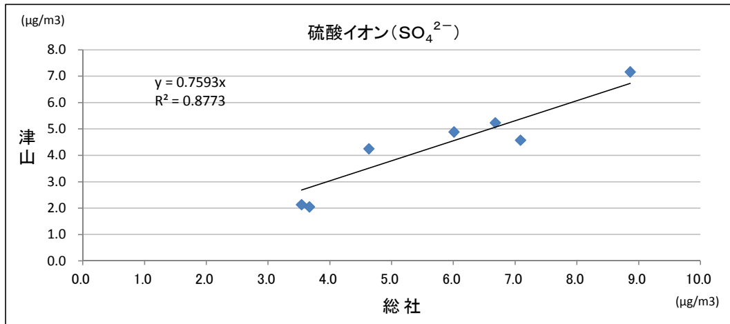
図11-1 (H25 冬季) 総社と津山における硫酸イオンの測定値比較
