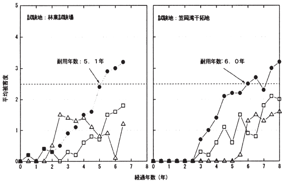
図 - 2 ヒノキ心材杭の被害経過 ● : 頂部、○ : 地際部、△ : 地中部
