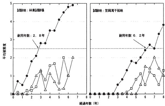
図 - 1 スギ心材杭の被害経過 ● : 頂部、○ : 地際部、△ : 地中部
