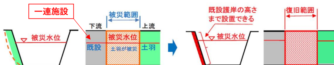
【図 5】 上下流一方に既設護岸（一連施設）あり → 既設護岸の高さ
