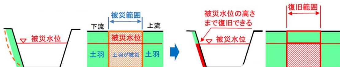
【図 3】 上下流に既設護岸なし → 被災水位
