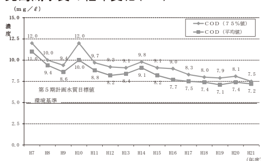
児島湖水質の経年変化(COD)
