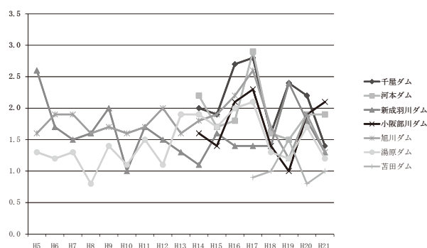
ダム湖水質経年変化(BOD:75%値)
