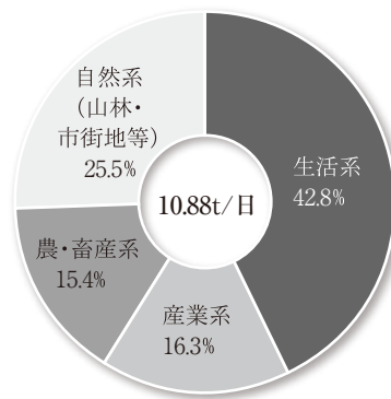
児島湖の平成20年度発生源別COD発生負荷量
