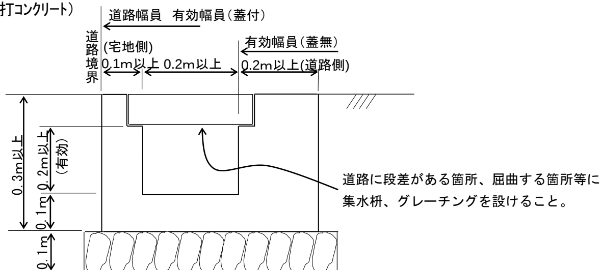
①U型側溝
