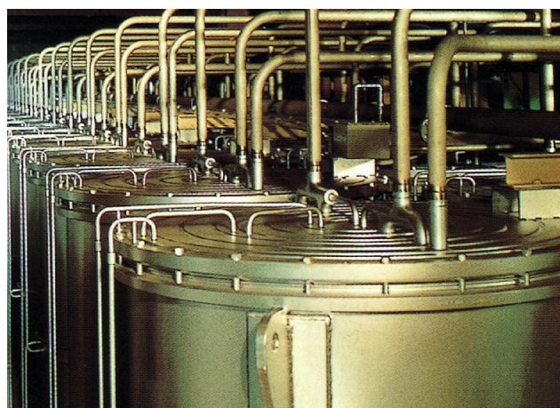
遠心分離機群（カスケード）
