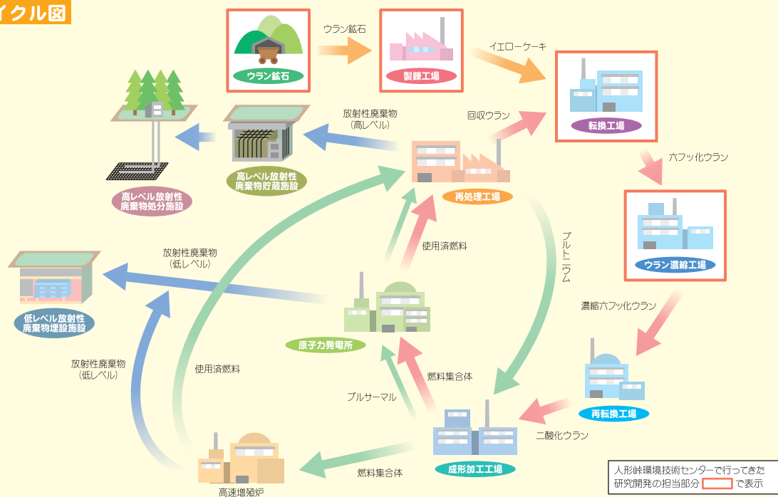
核燃料サイクル図
