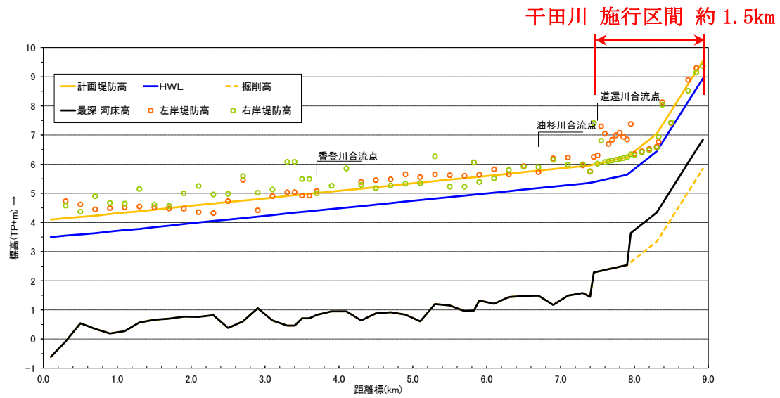
図-6(11) 干田川縦断面図
