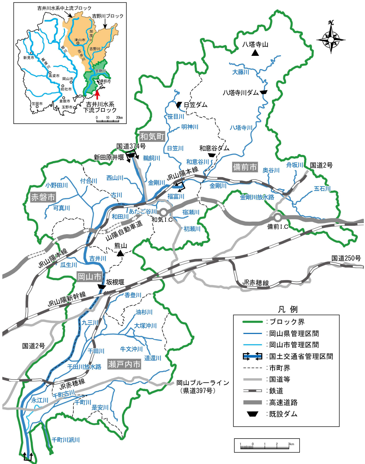
図ー1 吉井川水系下流ブロック概要図
