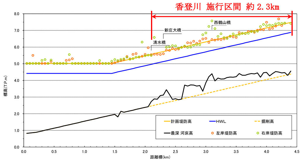
図-6(12) 香登川縦断面図
