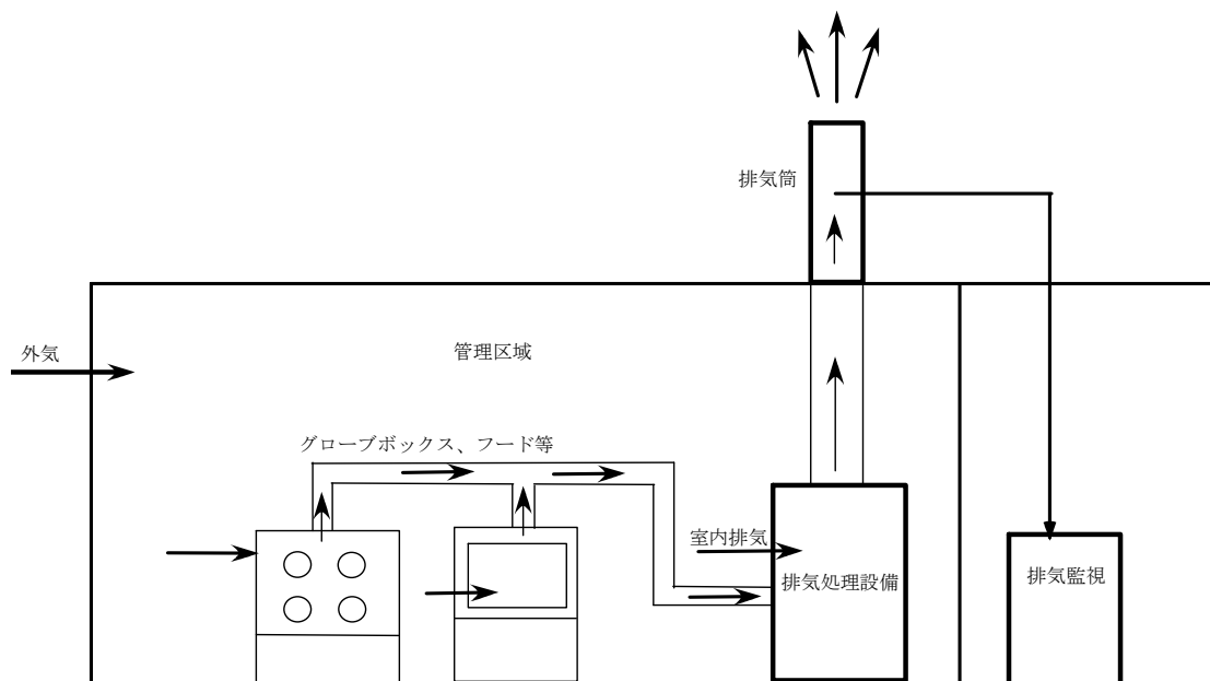
建屋排気系統図(イメージ)
