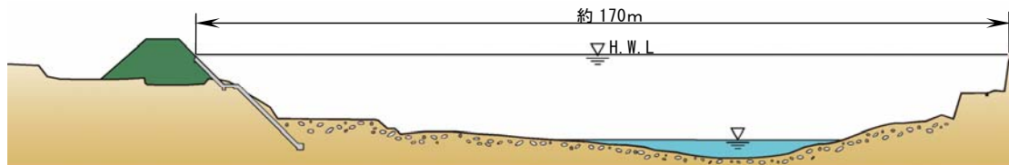
図－9 高梁川本川の代表断面図（宍粟地区から槻地区）
