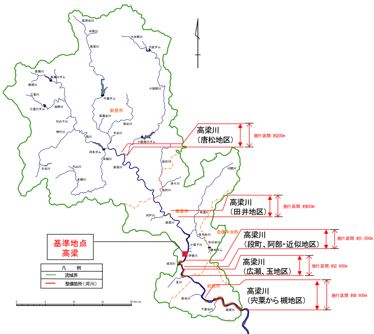
図-4 高梁川水系中上流ブロック 整備箇所位置
