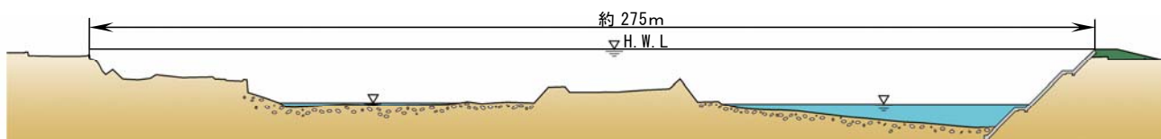
図－8 高梁川本川の代表断面図（宍粟地区から槻地区）
