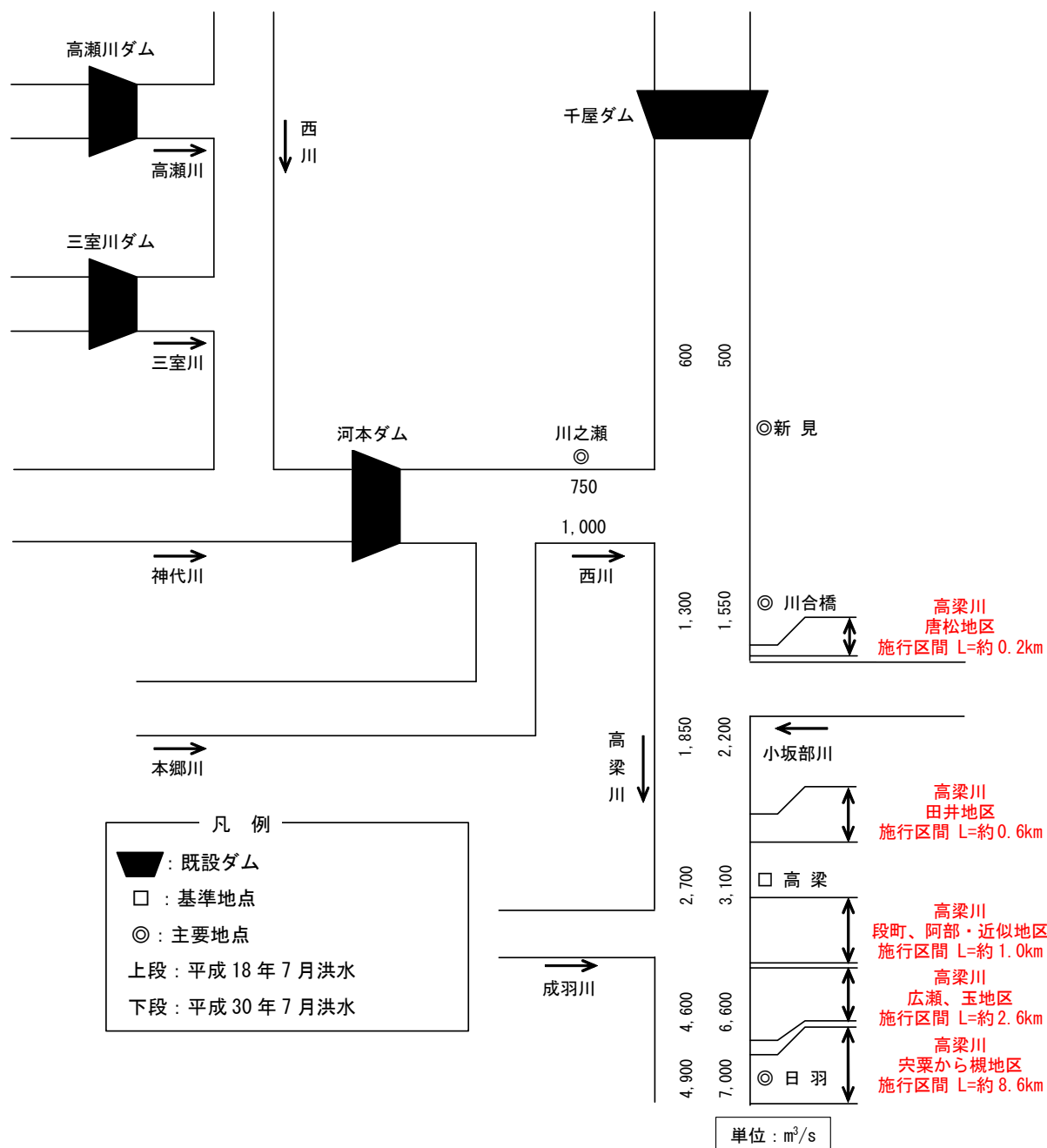
図ー6 高梁川水系中上流ブロックのH18.7洪水とH30.7洪水の流量配分図
