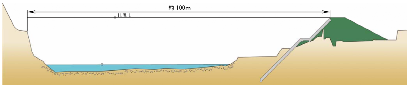
図－12 高梁川本川の代表断面図（田井地区）
