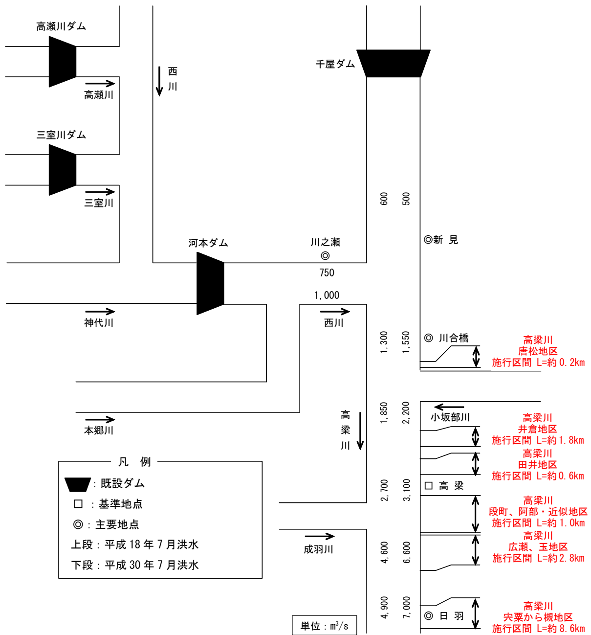
図-6 高梁川水系中上流ブロックの H18.7 洪水と H30.7 洪水の流量配分図
