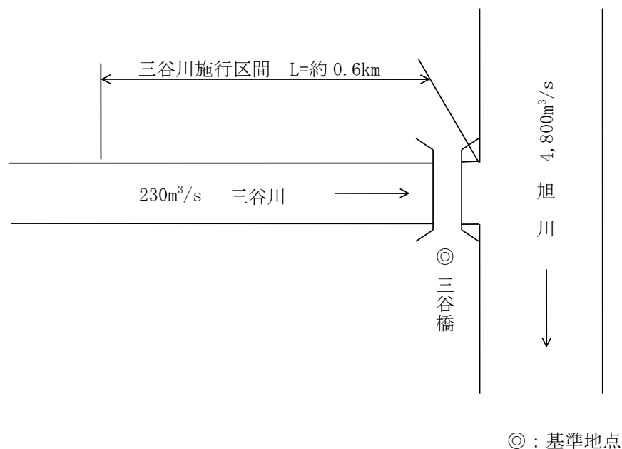
図 3-1-6 三谷川施行区間 整備計画目標流量配分図
