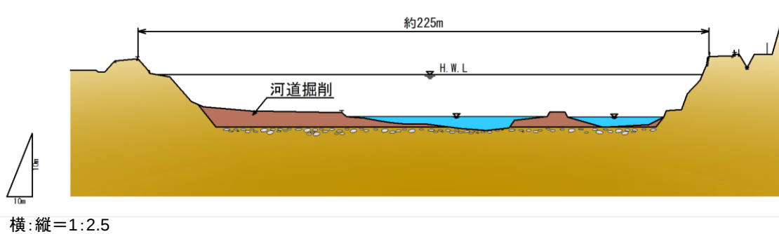
図 3-1-5 (3) 旭川本川施行区間（御津宇垣地区） 横断図 （28K800）
