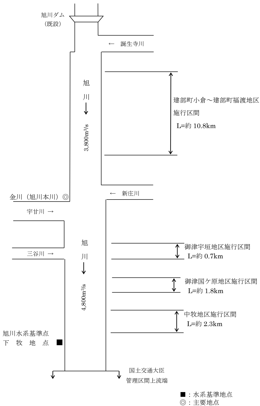
図 3-1-2 旭川本川施行区間 整備計画目標流量配分図
