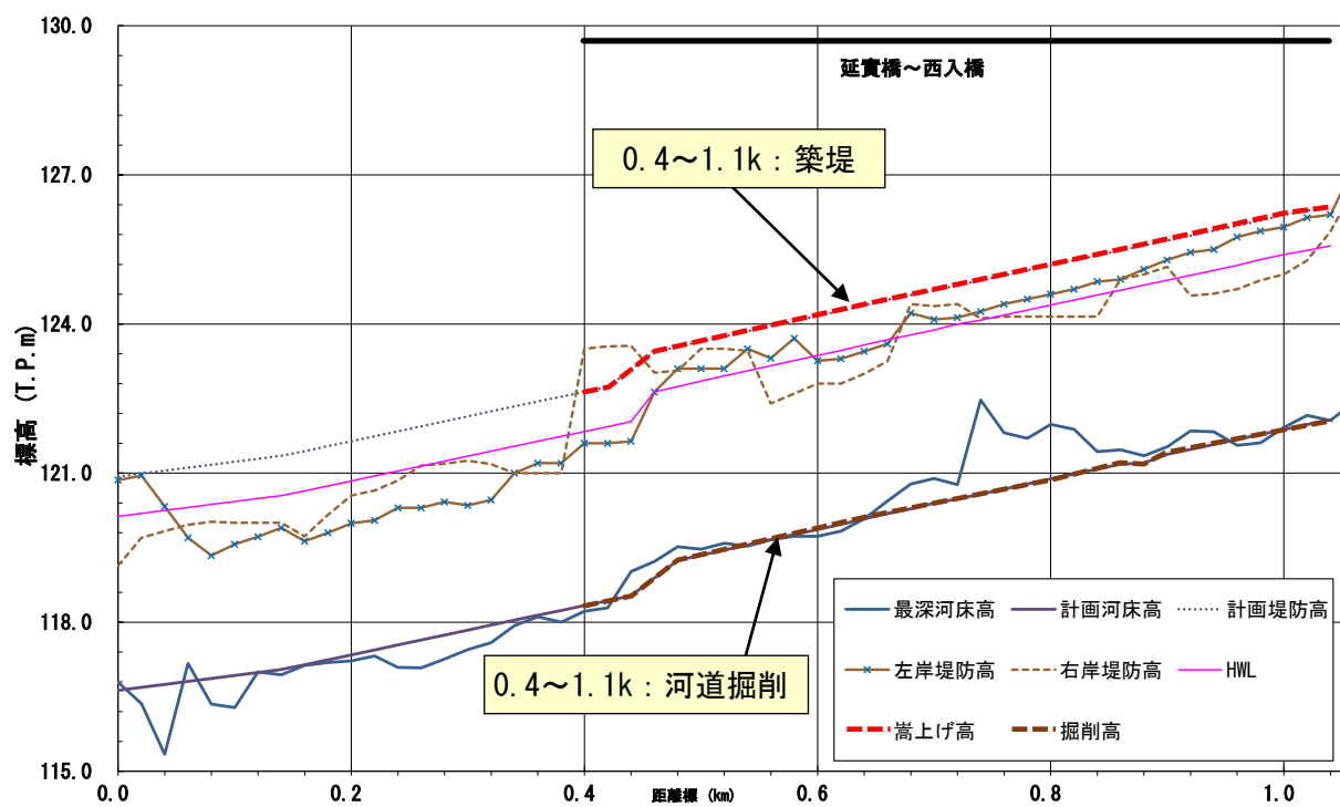
図 3-1-12 誕生寺川 縦断面図
