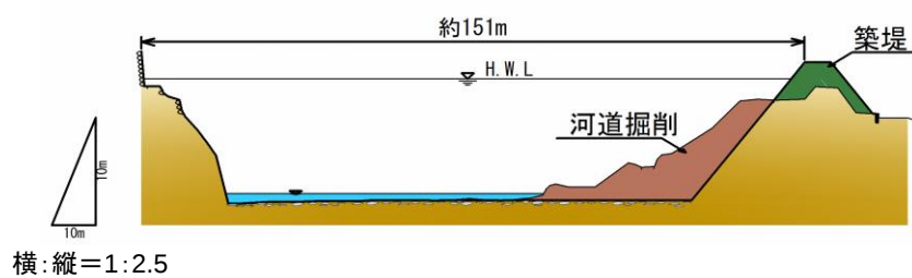
図 3-1-5 (1) 旭川本川施行区間（中牧地区） 横断図 （22K800）
