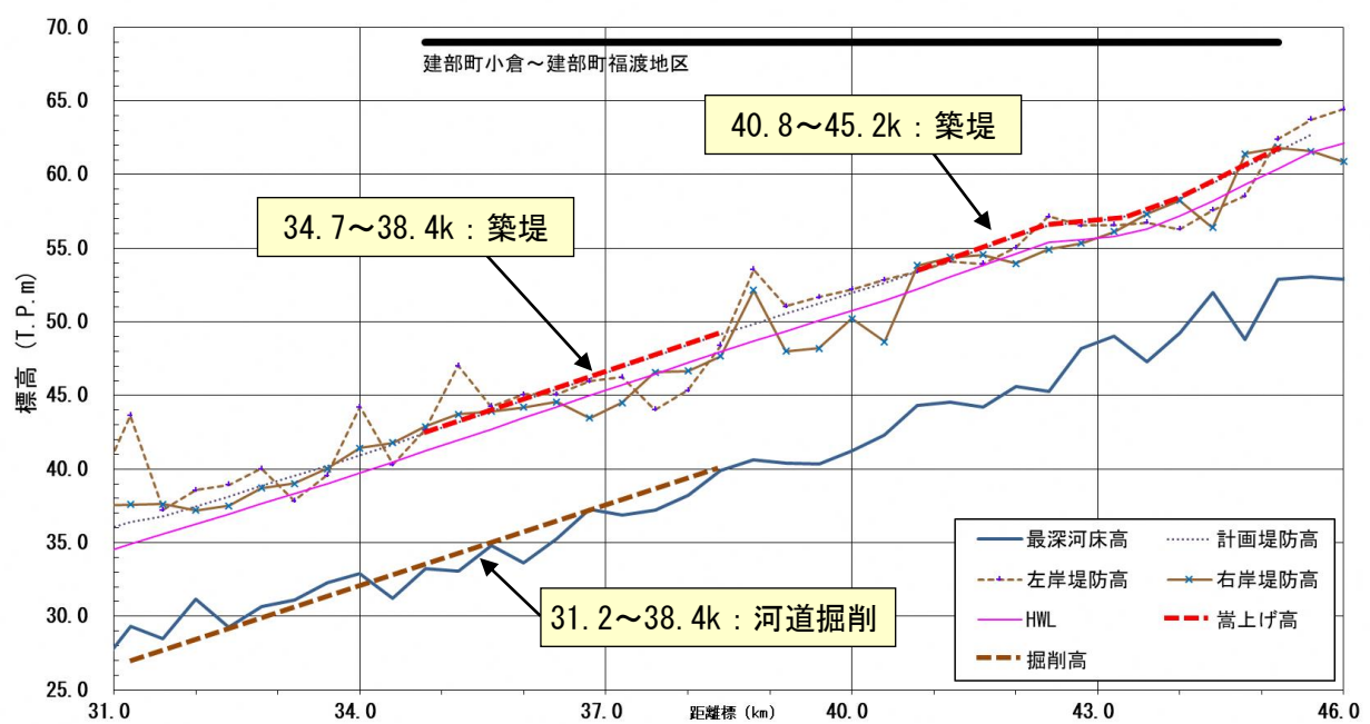
図 3-1-4 旭川本川 縦断図
