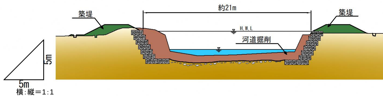
図 3-1-13 誕生寺川施行区間横断面図 (0k840) S=1:200
