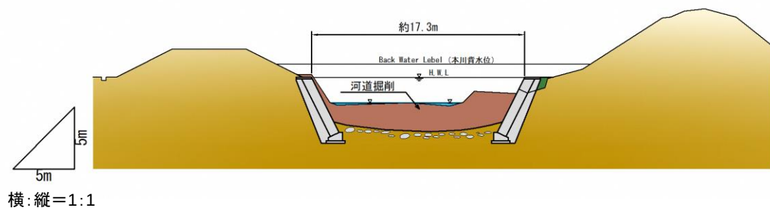
図 3-1-9 三谷川施行区間横断面図 (0k400)
