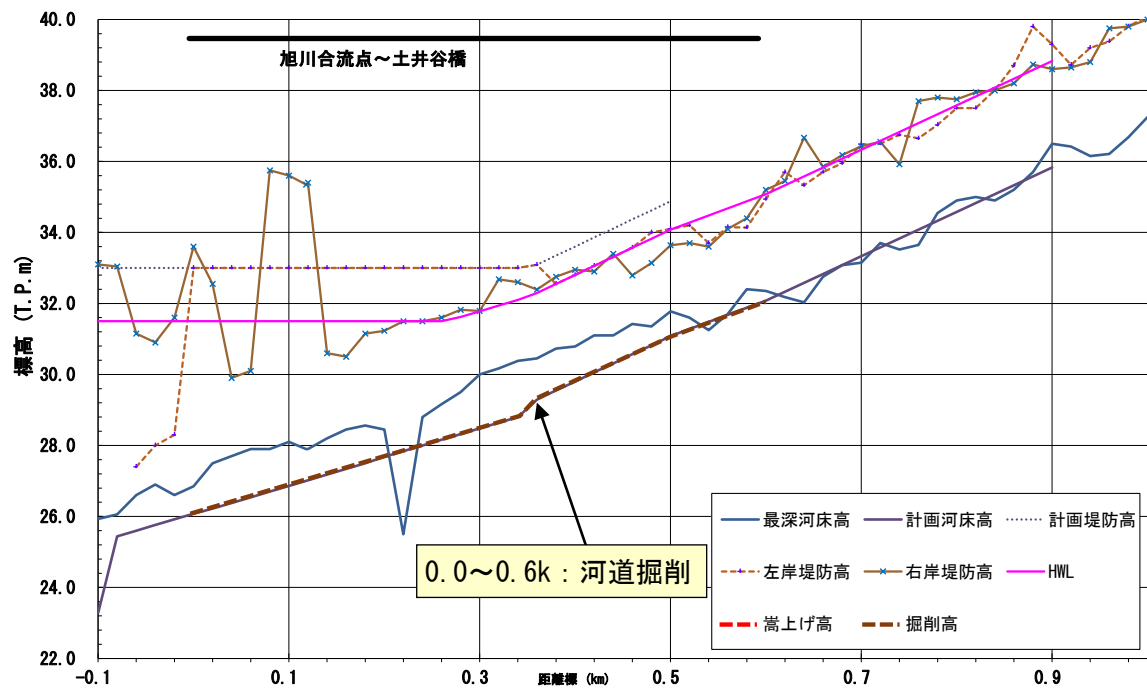
図 3-1-8 三谷川 縦断面図
