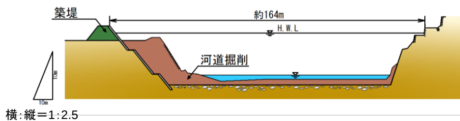
図 3-1-5 (2) 旭川本川施行区間（御津国ヶ原地区） 横断図 （26k800）
