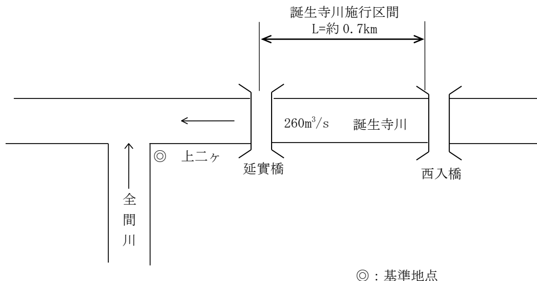
図 3-1-10 誕生寺川施行区間 整備計画目標流量配分図
