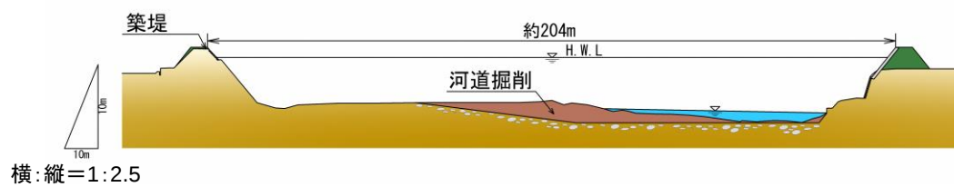
図 3-1-5 (4) 旭川本川施行区間（建部町小倉～建部町福渡地区） 横断図 （36K800）
